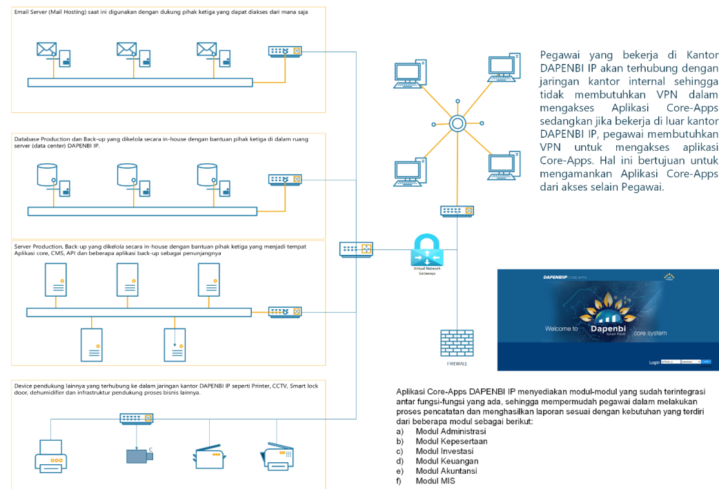
Gambar 2 Network Diagram DAPENBI IP
